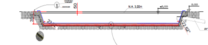
CORTE AA Esc.: 1/200
